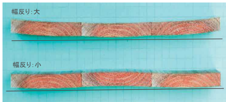
写真2 矧ぎ合わせ接着した板目板の収縮変形（木表・木裏の配置に注目）
