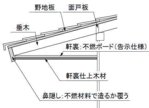
図 3.3 防火構造（30 分）
